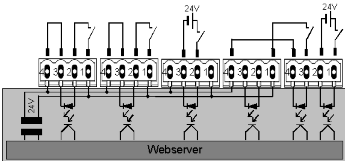
Abbildung 8.2.1b: Alternative Optokopplerbeschaltung.
