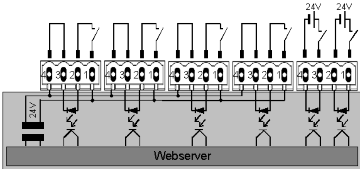
Abbildung 8.2.1a: Optokopplerbeschaltung.
